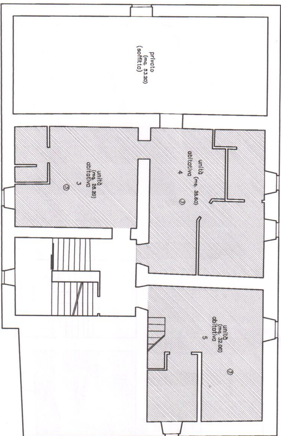
Pianta piano quarto
